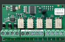
AUXI-R 01755 5 relaismodule
